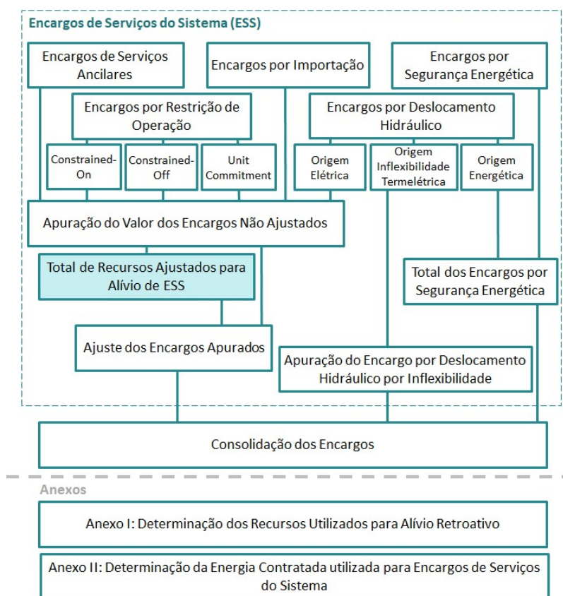
Figura 16: Esquema Geral do Módulo de Regras: "Encargos"
