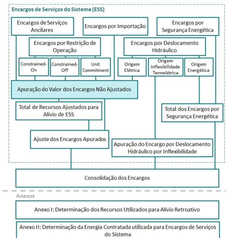
Figura 15: Esquema Geral do Módulo de Regras: “Encargos”
