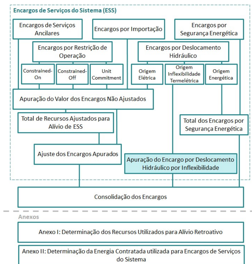
Figura 19: Esquema Geral do Módulo de Regras: “Encargos”
