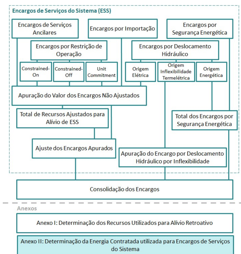
Figura 23: Esquema Geral do Módulo de Regras: “Encargos”
